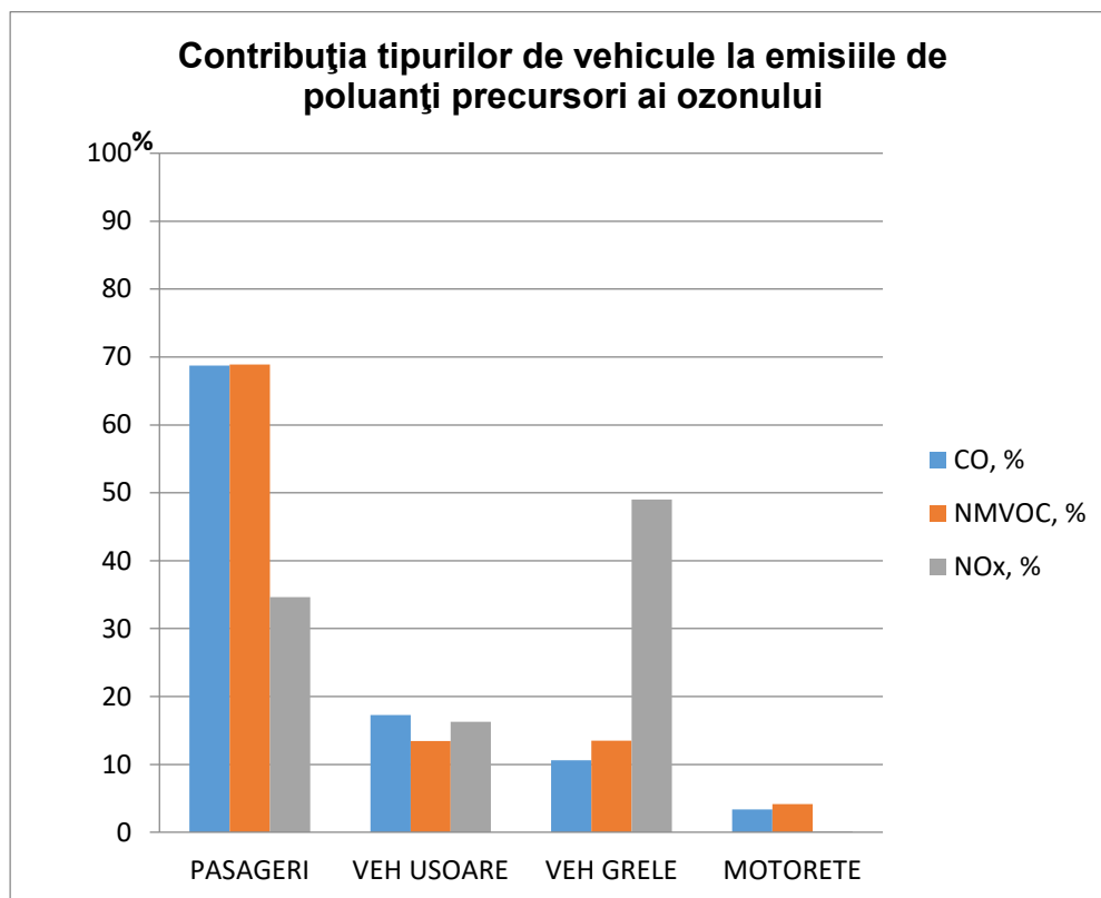
Figura I.2.1.3.3. Contribuția tipurilor de vehicule la emisiile de poluanți precursori ai ozonului în județul Buzău în anul 2019
