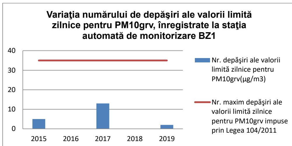
Fig. I.1.1.3.1. Variația numărului de depășiri ale valorii limită zilnice pentru PM10grv, stația BZ-1
