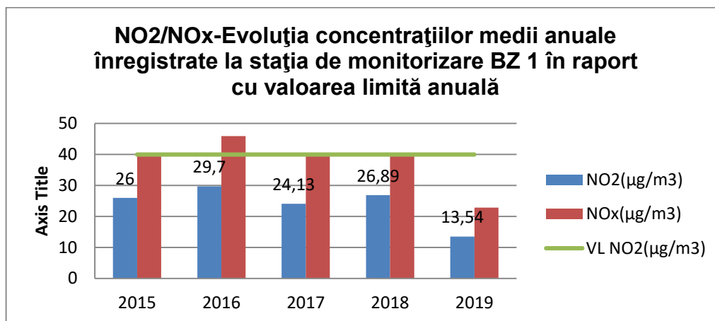
Fig. I.1.1.2.1.1. Evoluția concentrațiilor medii anuale NO 2 /NO x la stația BZ1
