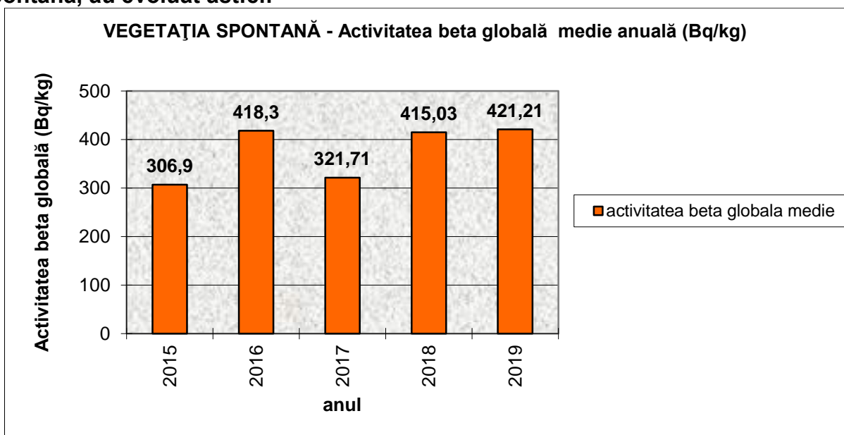
Fig. IX.1.4.2. Activitatea specifică beta globală medie anuală pentru vegetația spontană, comparativ în perioada 2015-2019
