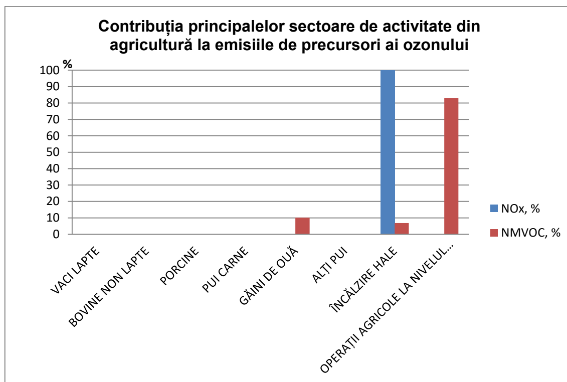
Figura I.2.1.4.2. Contribuția principalelor sectoare de activitate din agricultură la emisiile de precursori ai ozonului în 2019
