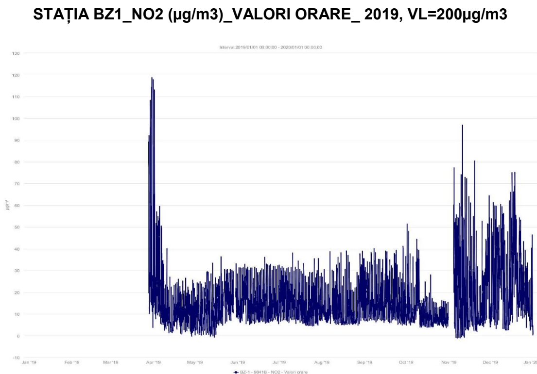
Figura I.1.1.1.1.2. Concentrații medii orare de NO 2 la stația BZ-1 în anul 2019
