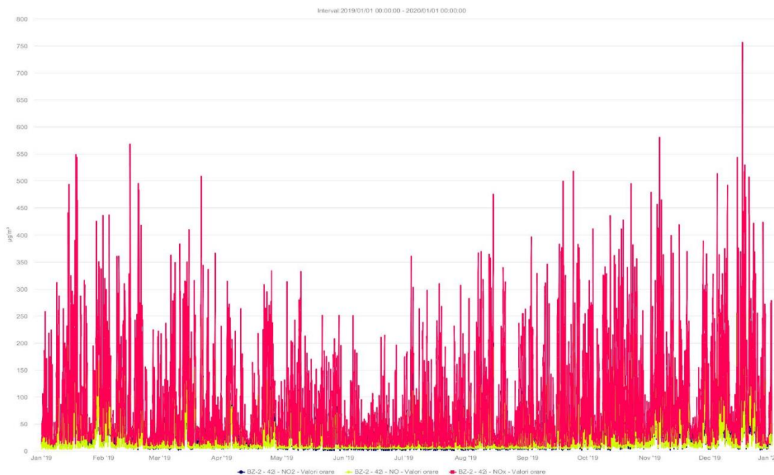
Fig. I.1.1.1.5. Variația concentrațiilor medii orare pentru NO 2 /NO x /NO la stația de monitorizare BZ2, în anul 2019
