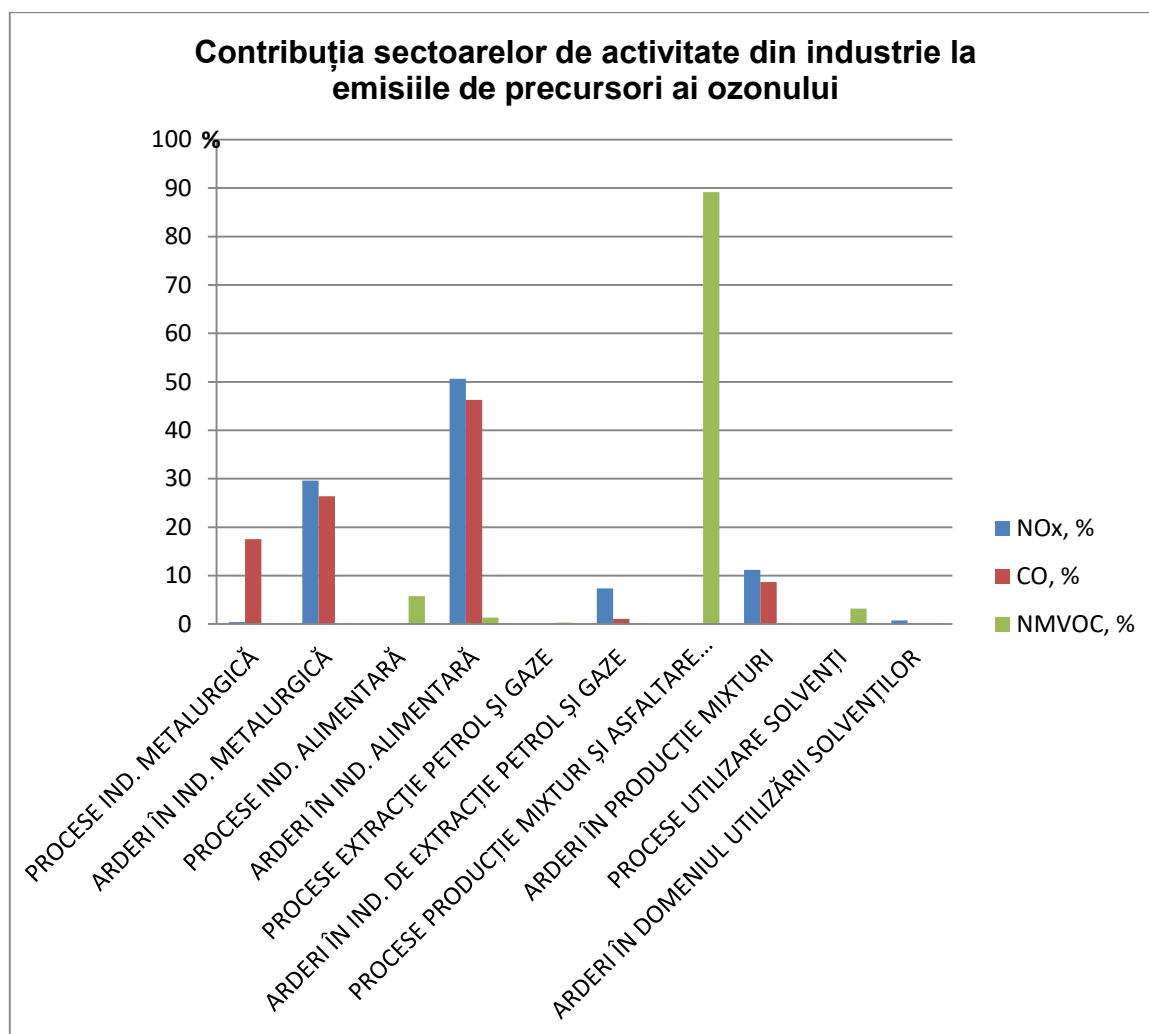
Figura I.2.1.2.5. Contribuția sectoarelor de activitate din industrie la emisiile de precursori ai ozonului
