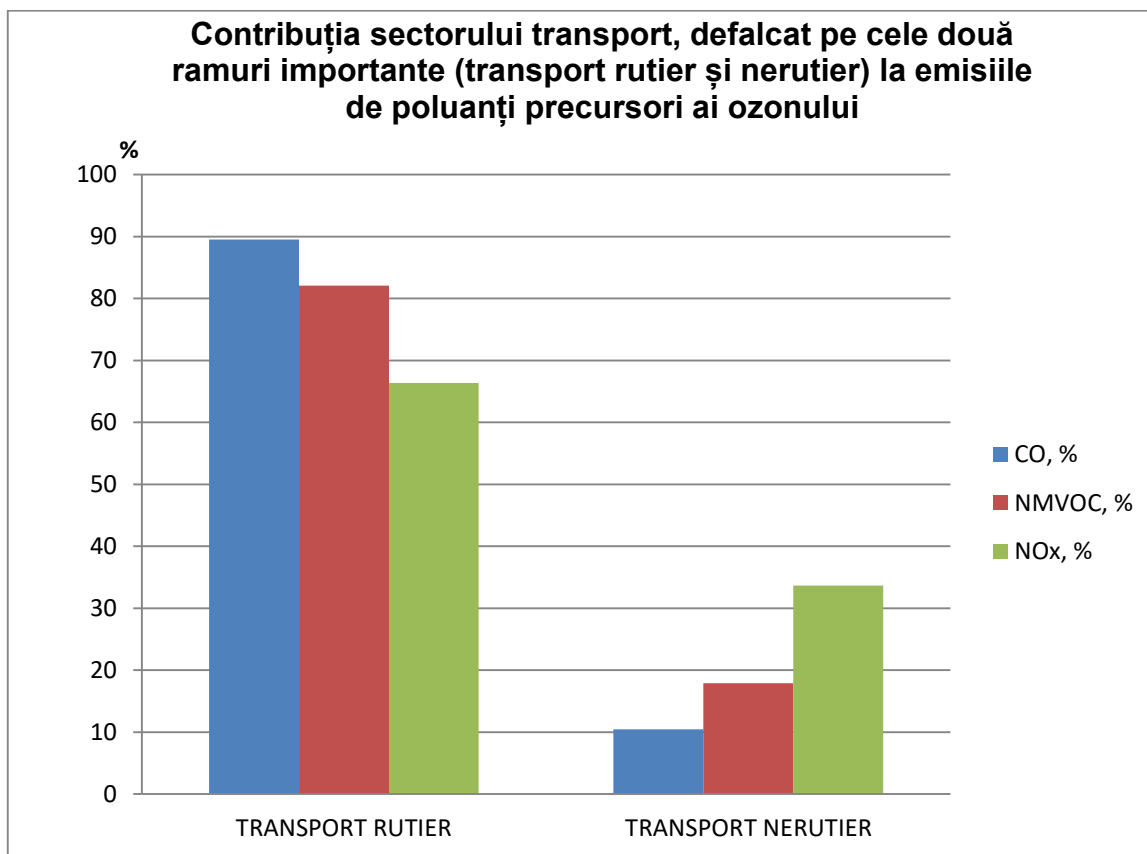
Figura I.2.1.3.4. Contribuția sectorului transport, defalcat pe cele două ramuri importante (transport rutier și transport nerutier) la emisiile de poluanți precursori ai ozonului în județul Buzău în anul 2019
