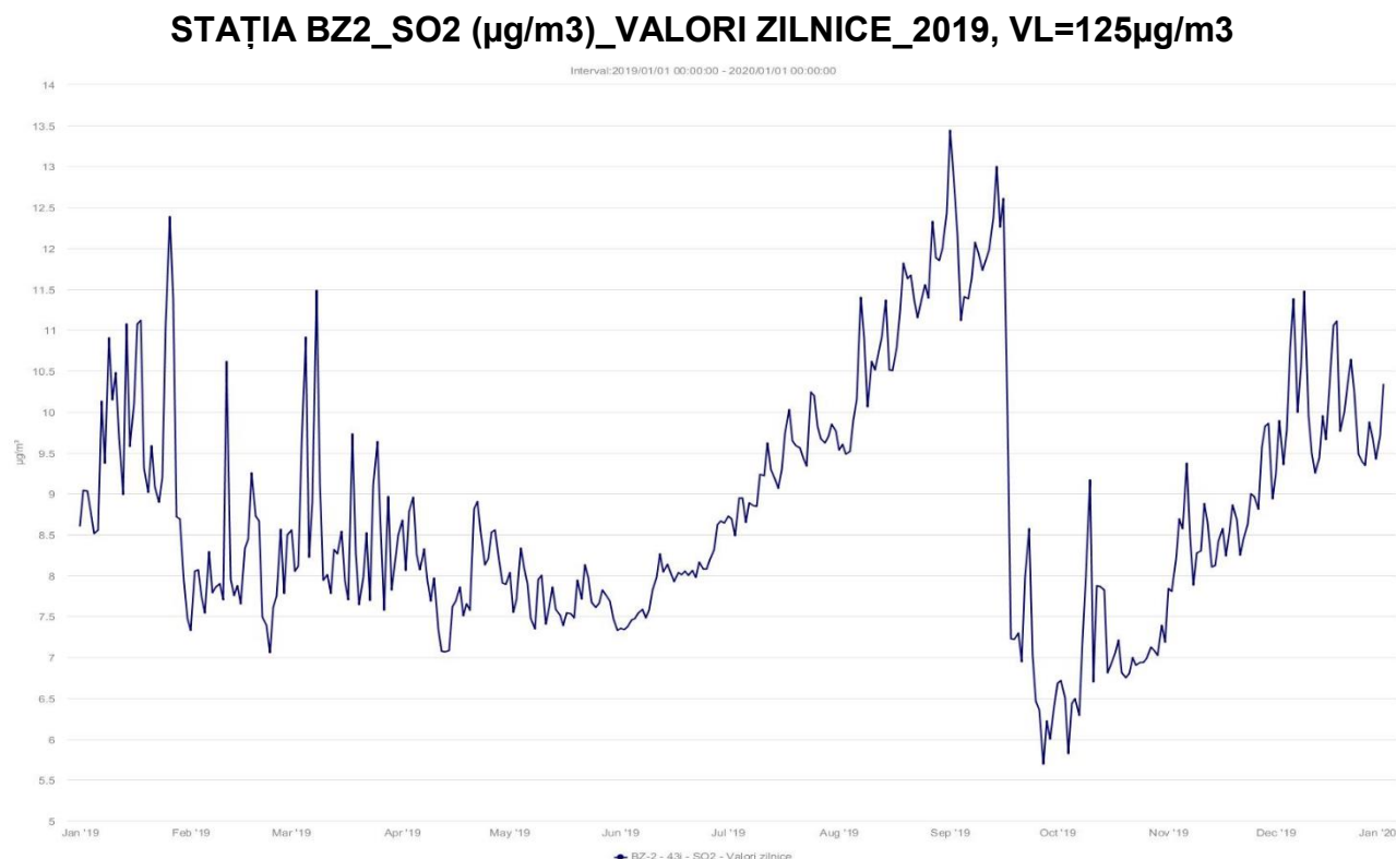
Fig. I.1.1.1.2.5. SO 2 concentrații medii zilnice la stația BZ-1 în anul 2019
