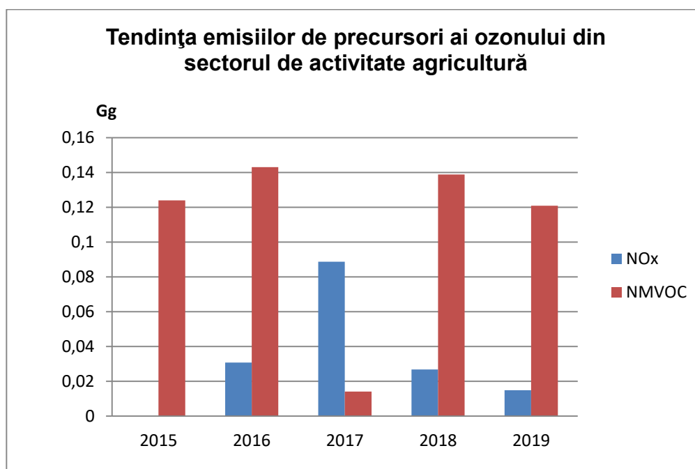
Figura I.3.1.10. Tendința emisiilor de poluanți precursori ai ozonului din agricultură
