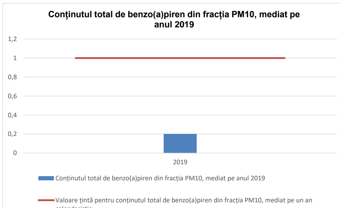
Fig. I.1.1.1.7.2. Conținut total de benzo(a)piren din fracția PM10 mediat pentru anul 2019 în municipiul Buzău
