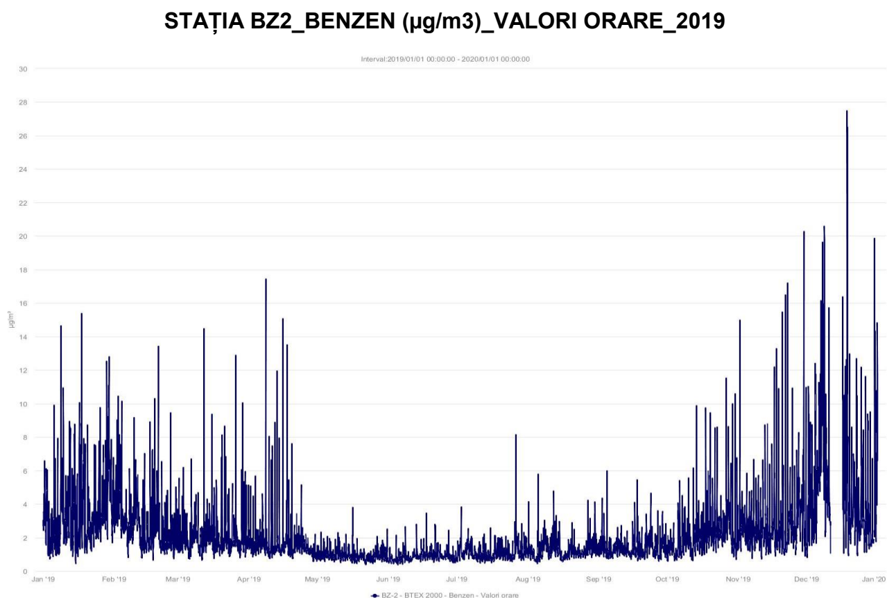
Fig. I.1.1.1.5.2. Variația concentrațiilor medii orare pentru benzen la stația BZ2 în anul 2019
