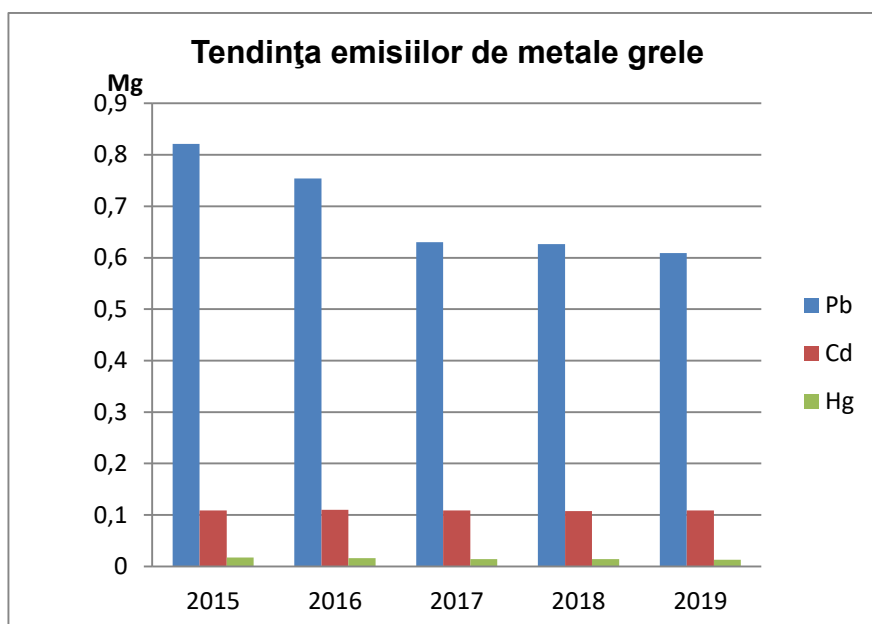
Figura I.3.1.16. Tendința emisiilor totale de metale grele
