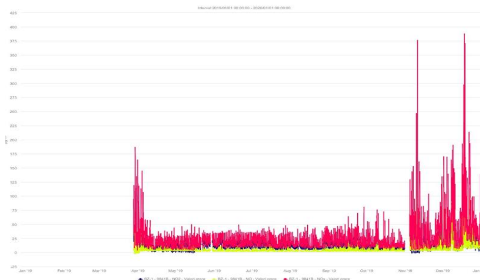
Fig. I.1.1.1.3. Variația concentrațiilor medii orare pentru NO 2 /NO x /NO la stația de monitorizare BZ1, în anul 2019
