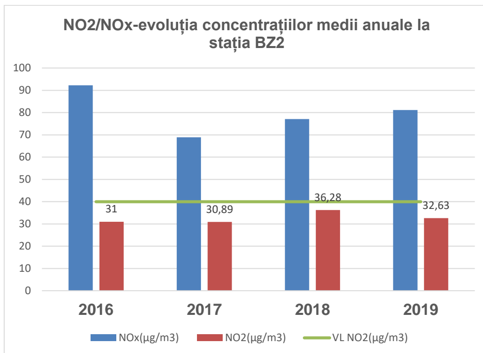
Fig. I.1.1.2.1.2. Evoluția concentrațiilor medii anuale de NO2/ NOx la stația BZ2
