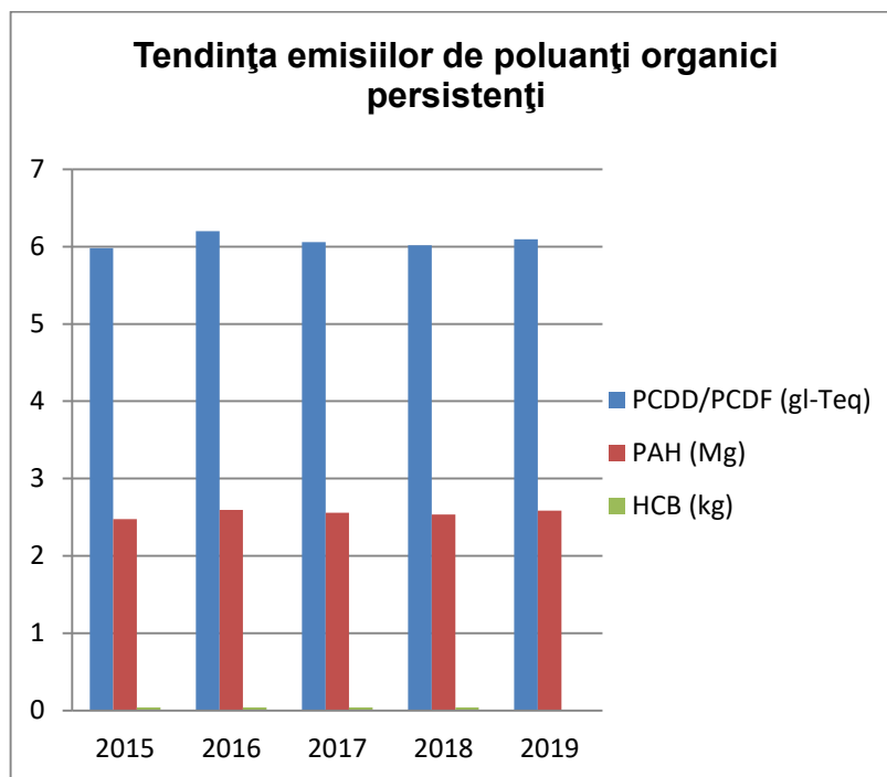
Figura I.3.1.20. Tendinta emisiilor totale de poluanți organici persistenți
