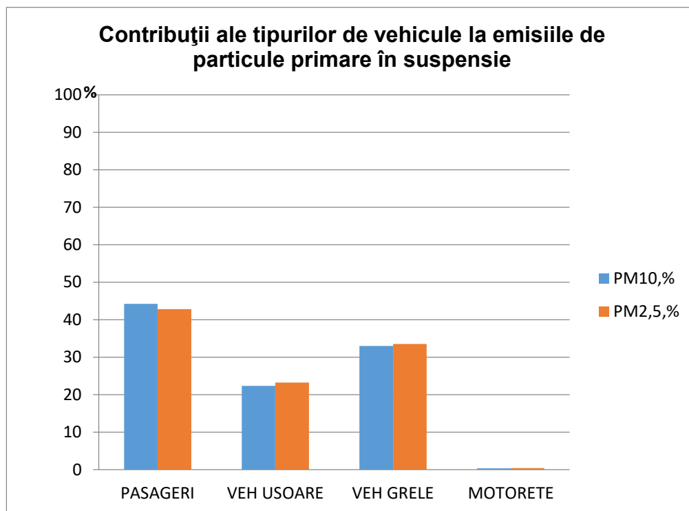
Figura I.2.1.3.5. Contribuția tipurilor de vehicule la emisiile de particule primare și precursori secundari de particule în județul Buzău în anul 2019
