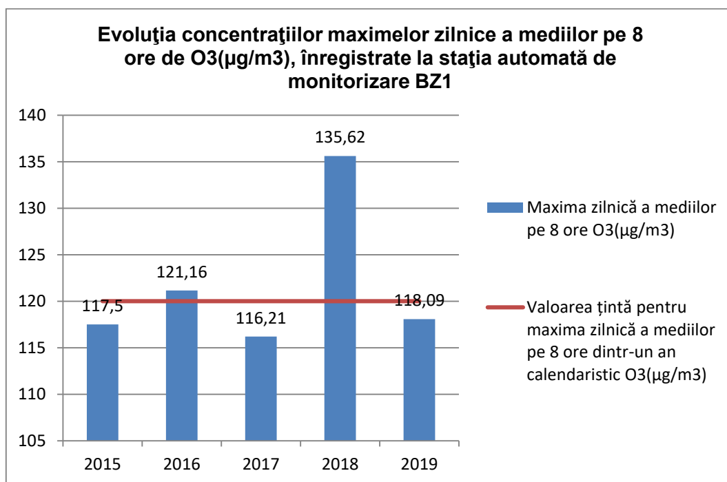
Fig. I.1.1.2.6.1. Evoluția concentrațiilor maximelor zilnice a mediilor pe 8 ore dintr-un an calendaristic de O 3
