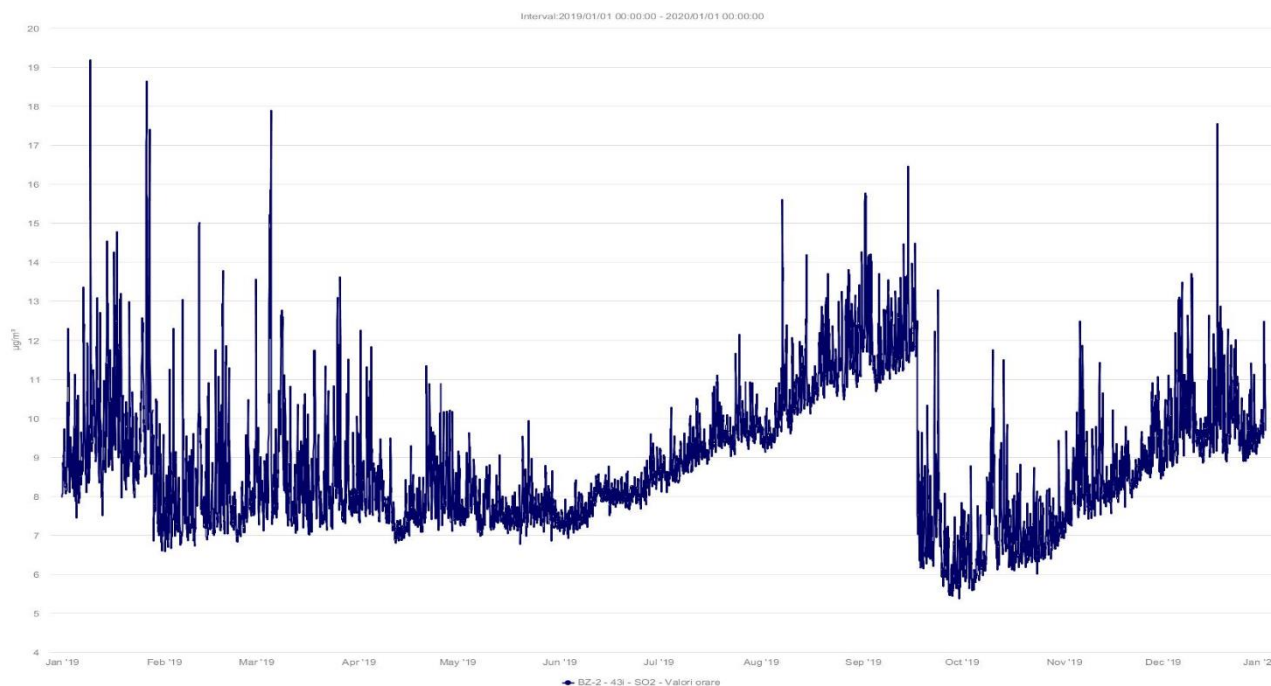
Fig. I.1.1.1.2.4. SO2 concentrații medii orare la stația BZ-2, în anul 2019
