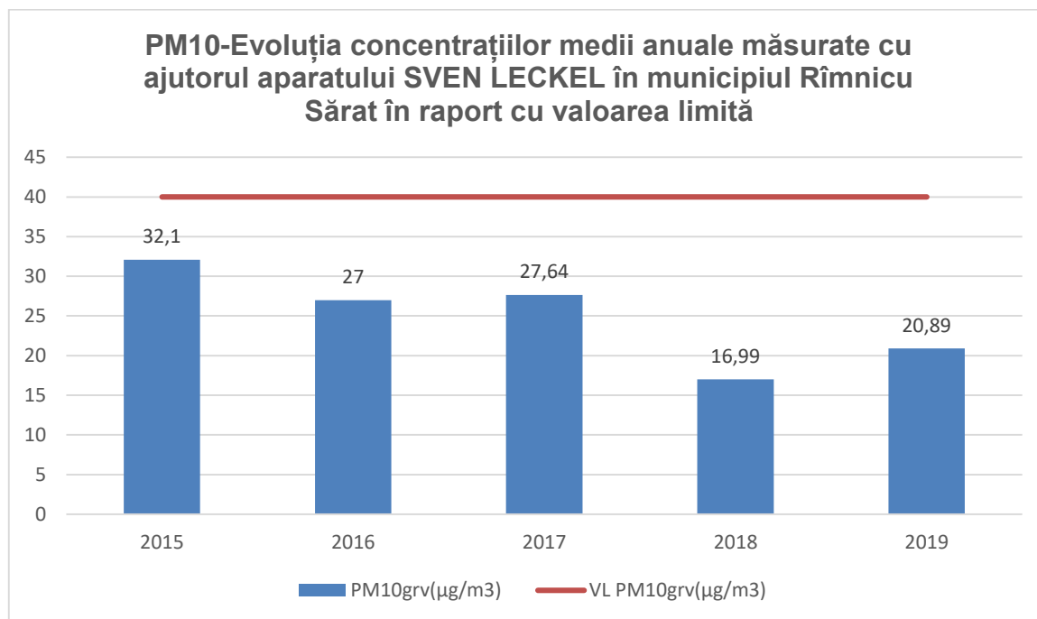
Fig. I.1.1.2.3.1.3. Evoluția concentrațiilor medii anuale PM10 – SVEN LECKEL
