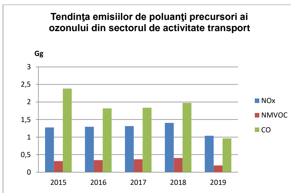
Figural.3.1.9. Tendința emisiilor de poluanți precursori ai ozonului din transport
