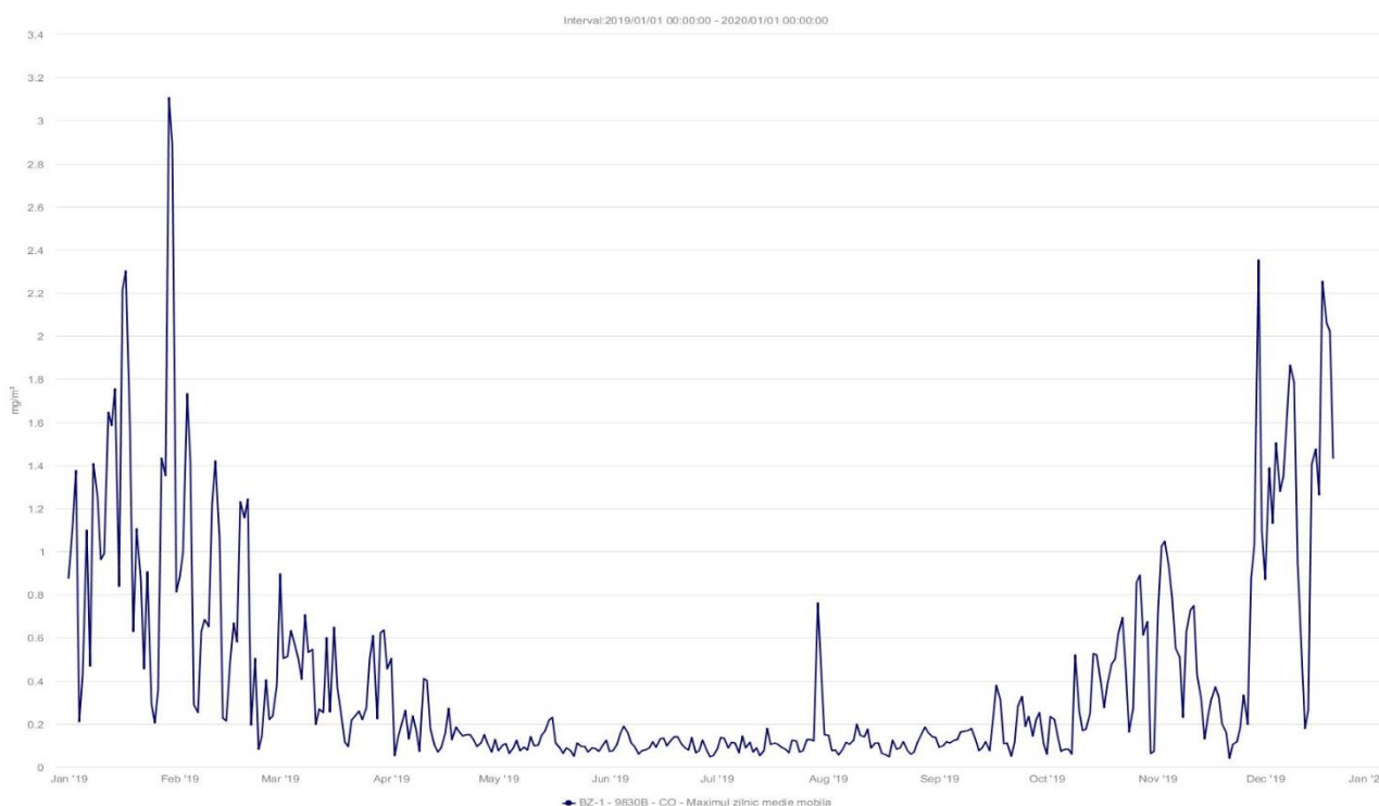
Fig. I.1.1.1.4.2. CO(mg/m3), Maxima zilnică a mediilor pe 8h în anul 2019 la stația BZ1
