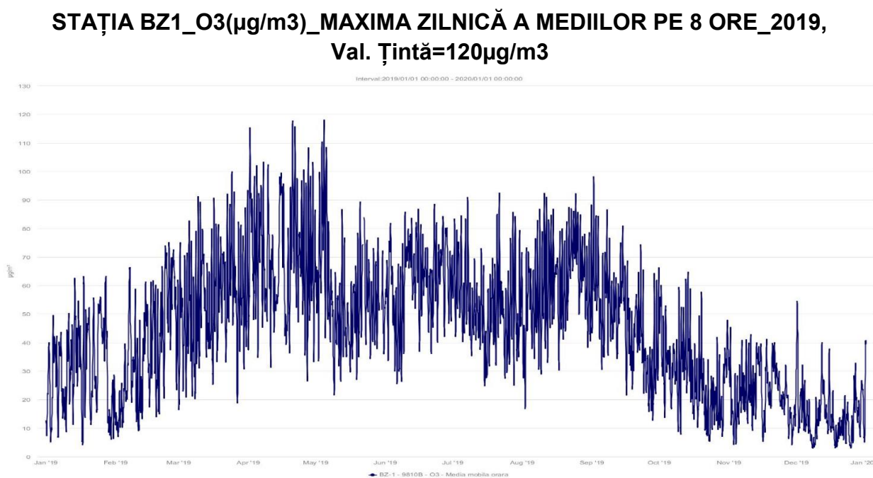
Fig. I.1.1.1.6.1. O3( \mu g/m 3 )-Maxima zilnică a mediilor pe 8h la stația BZ1, în anul 2019 Stația BZ-2, fiind de trafic, nu monitorizează ozonul.
