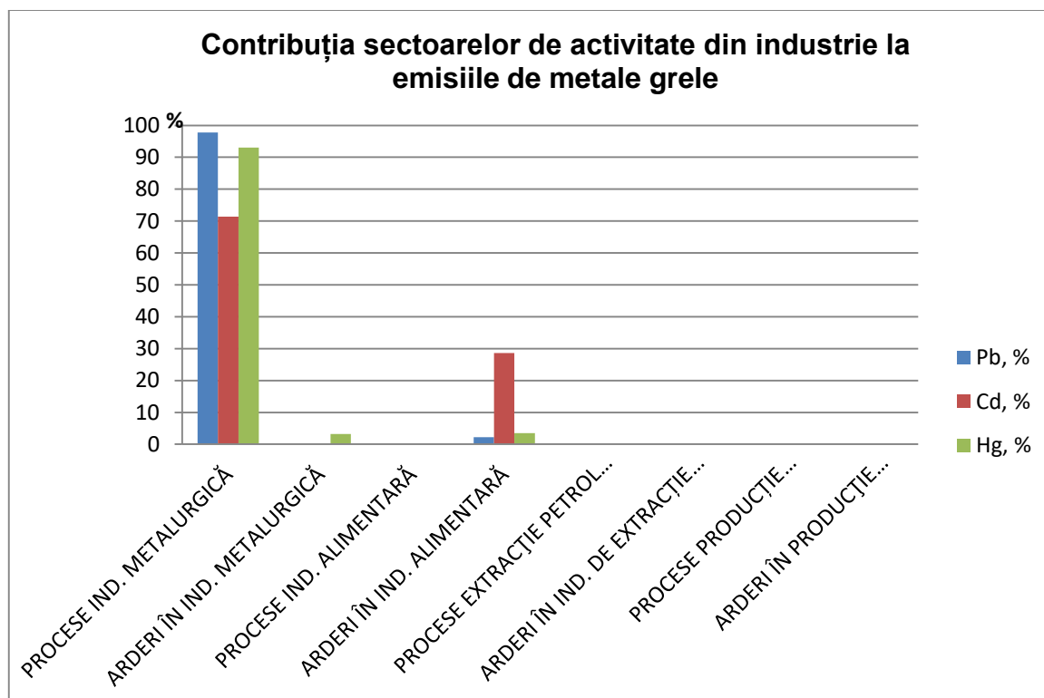
Figura I.2.1.2.9. Contribuția sectoarelor de activitate din industrie la emisiile de metale grele
