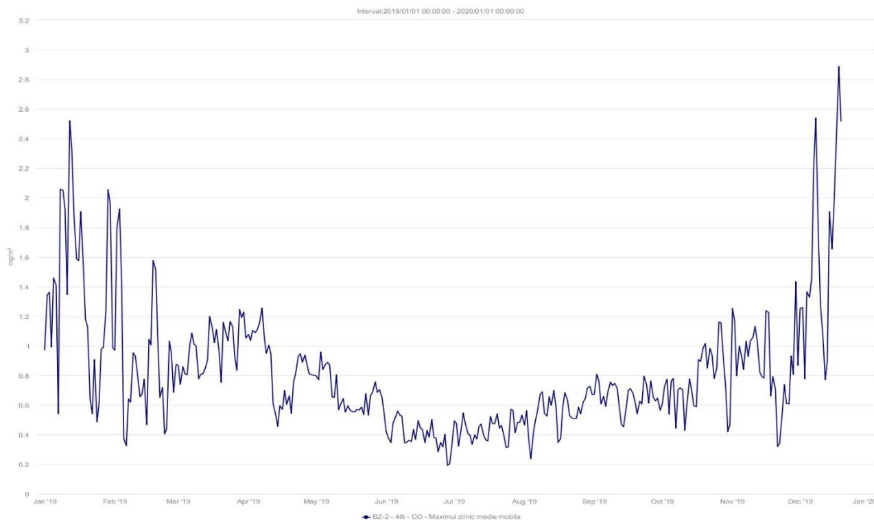
Fig. I.1.1.1.4.3. CO(mg/m3), Maxima zilnică a mediilor pe 8h în anul 2019 la stația BZ2
