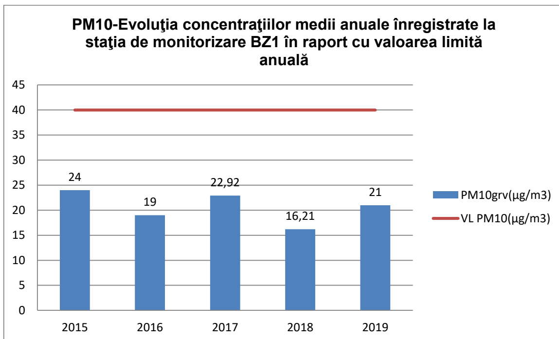
Fig. I.1.1.2.3.1.1. Evoluția concentrațiilor medii anuale PM10
