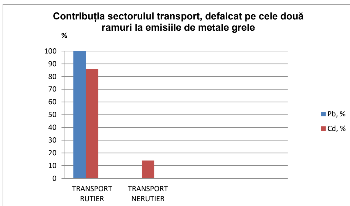
Figura I.2.1.3.8. Contribuția sectorului transport, defalcat pe cele două ramuri importante (transport rutier și transport nerutier) la emisiile de metale grele în județul Buzău în anul 2019
