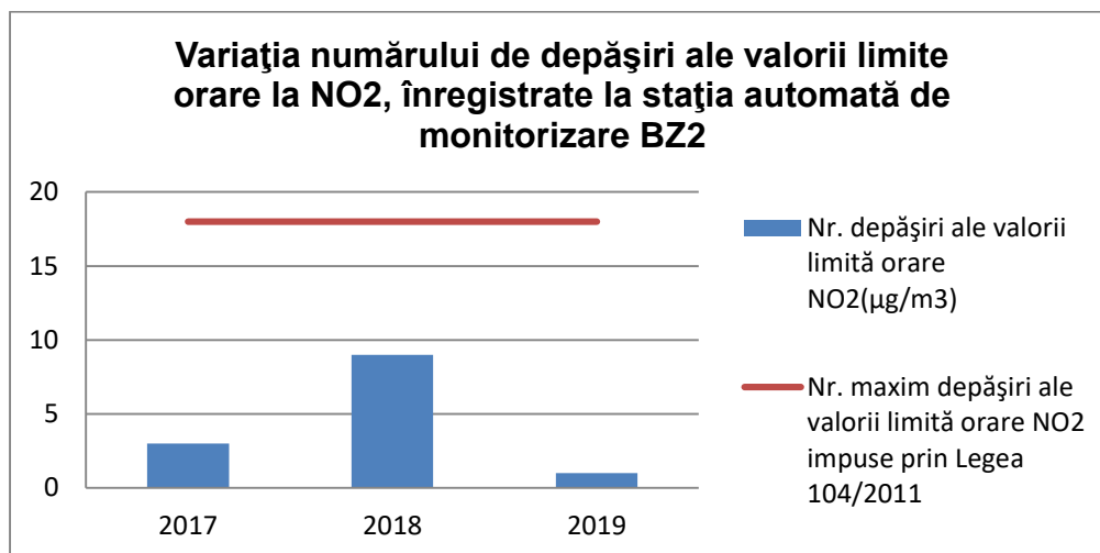
Fig. I.1.1.3.3. Variația numărului de depășiri ale valorii limite orare la NO2, stația BZ-2
