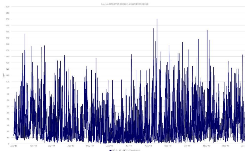
Figura I.1.1.1.4. Concentrații medii orare de NO 2 la stația BZ-2 în anul 2019
