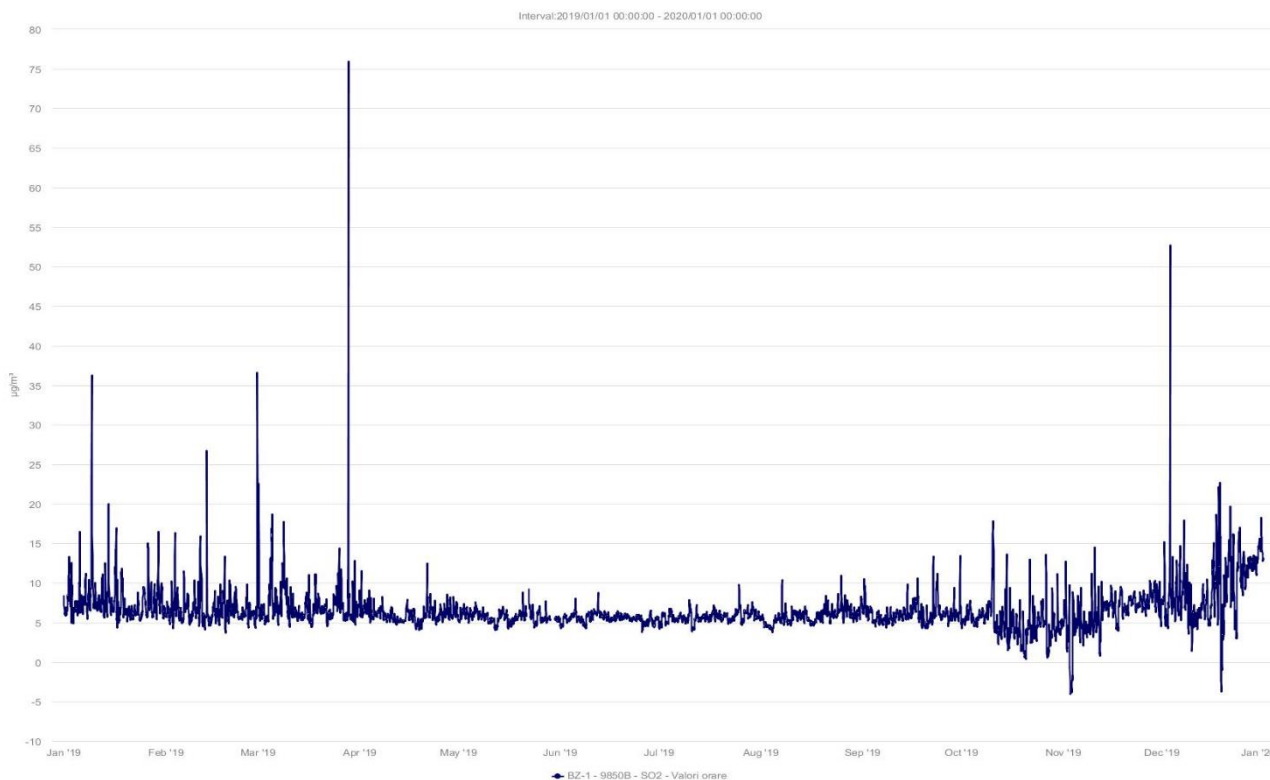
Fig. I.1.1.1.2.2. SO2 concentrații medii orare la stația BZ-1, în anul 2019
