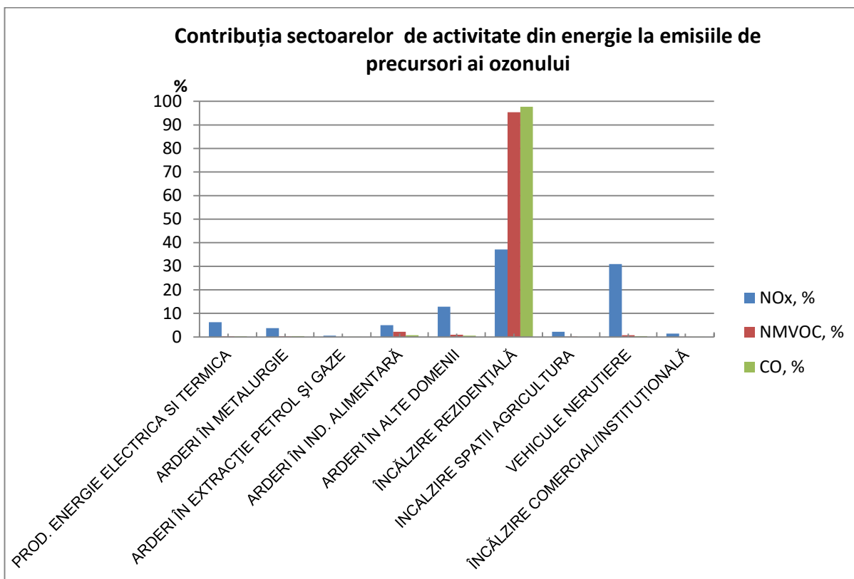
Figura 1.2.1.1.2. Contribuția sectoarelor de activitate din energie la emisiile de precursori ai ozonului
