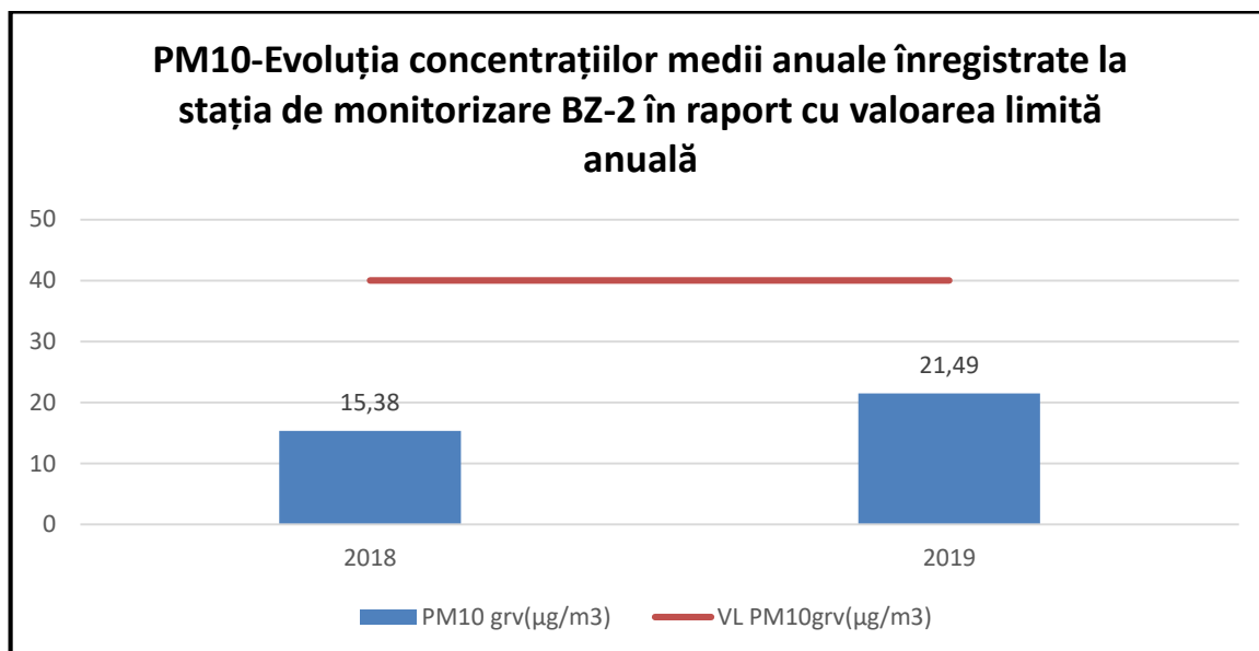
Fig. I.1.1.2.3.1.2. Evoluția concentrațiilor medii anuale de PM10 la stația BZ2
