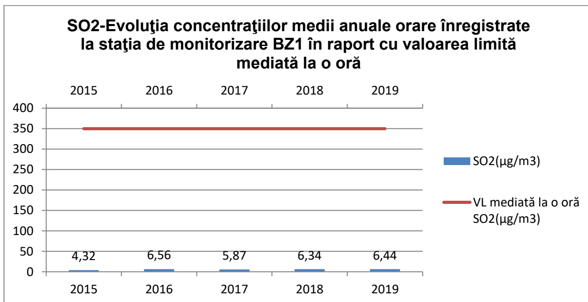
Fig. I.1.1.2.2.1. Evoluția concentrațiilor medii anuale orare de SO 2 la stația BZ1
