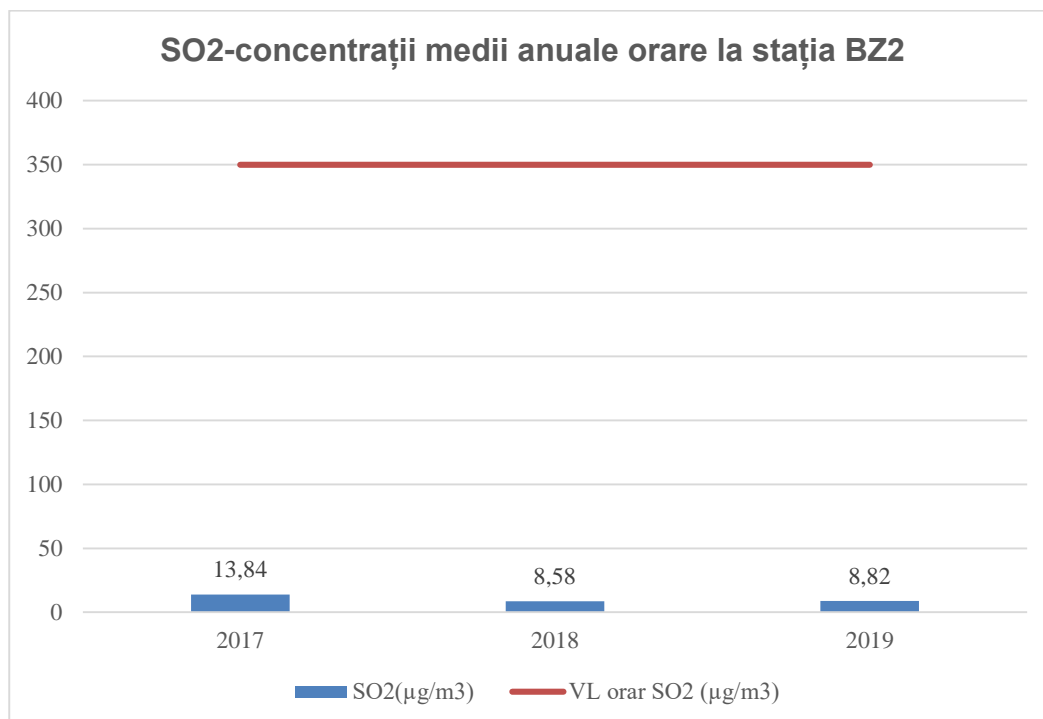
Fig. I.1.1.2.2.2. Evoluția concentrațiilor medii anuale orare de SO2 la stația BZ2
