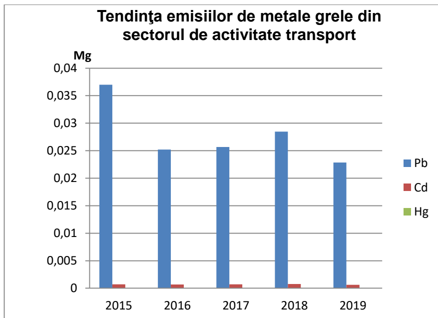
Figura I.3.1.19. Tendința emisiilor de metale grele din transport
