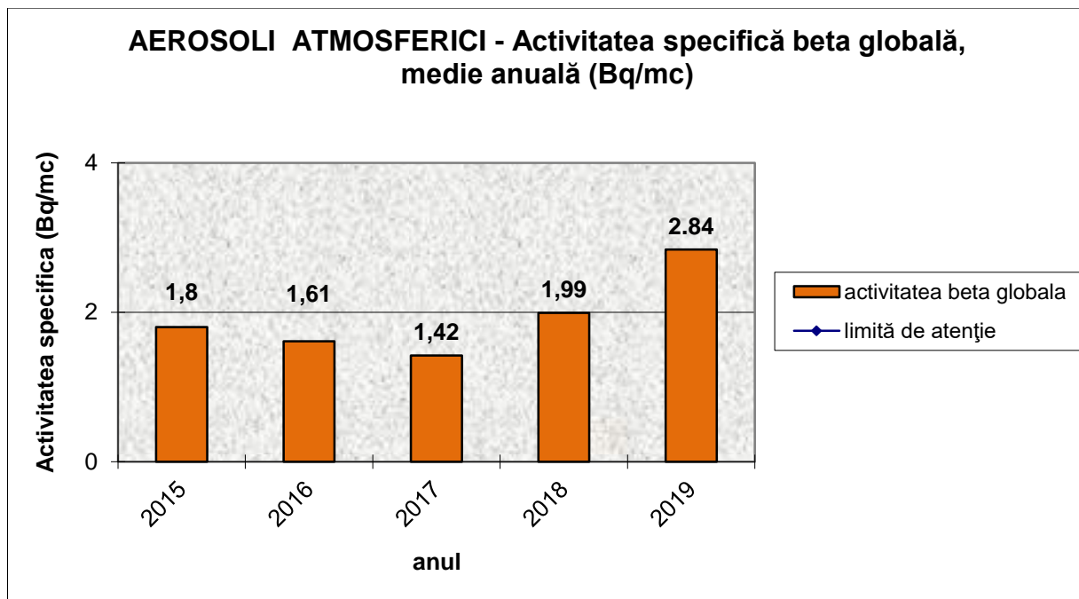
Fig. IX.1.1.2. Activitatea specifică beta globală medie anuală pentru aerosoli atmosferici (valori imediate), comparativ cu perioada 2015 - 2019
