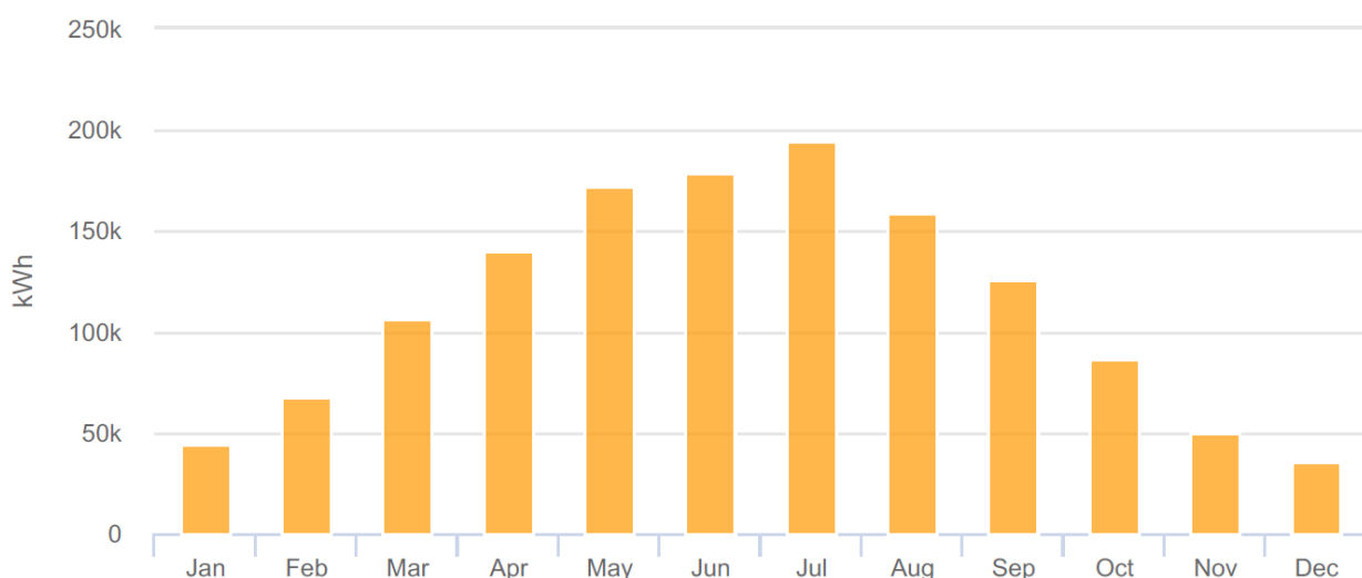
Fig.1 – cantitatea de energie electrica produsa (kWp/luna) – simularile au fost realizate cu programul HelioScope
